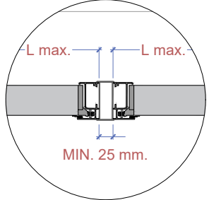
Sección planta con montante central (Solo sección persiana orientada 90° y guías)
