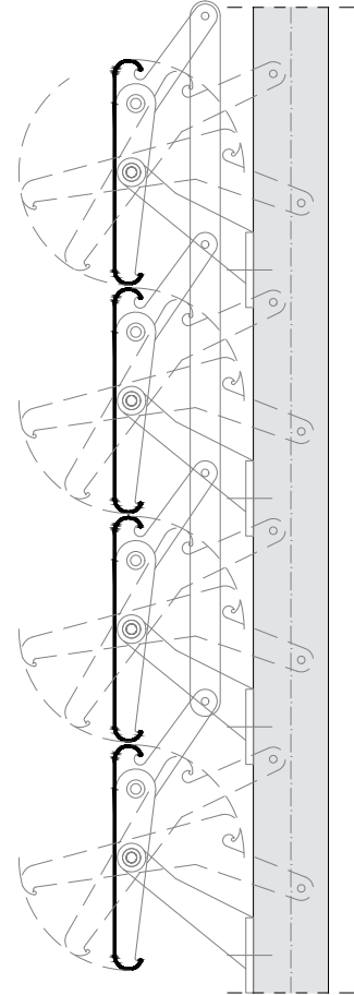
C 150 - orientable
